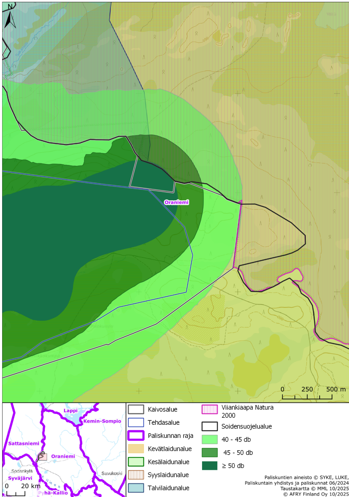
Kuva 5-2. Lähikuva melun leviämisalueesta tehdasalueen itäreunalla, kun työvaihe on lähimpänä Natura 2000 -suojelualueen rajaa. Kartalla esitetty kaivoksen maanpäällisen tehdasalueen itäreunaa.
