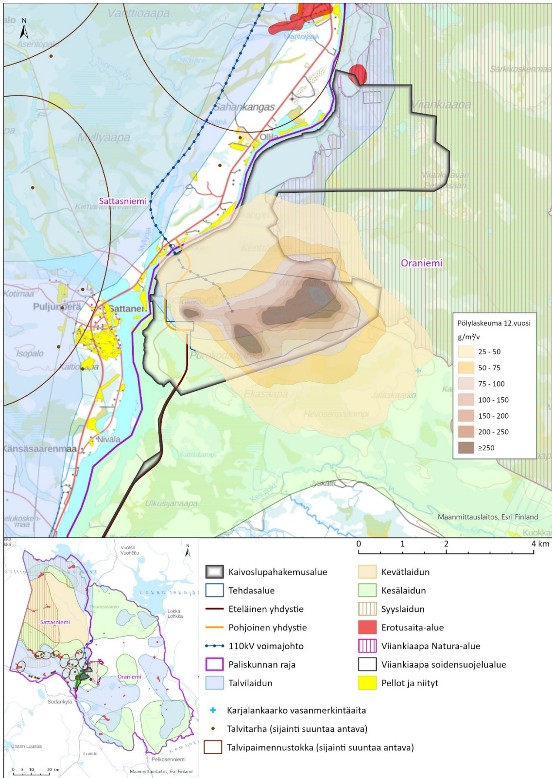
Kuva 5-10. Pölylaskeuman vuosikeskiarvo tuotantovuosi 12.
