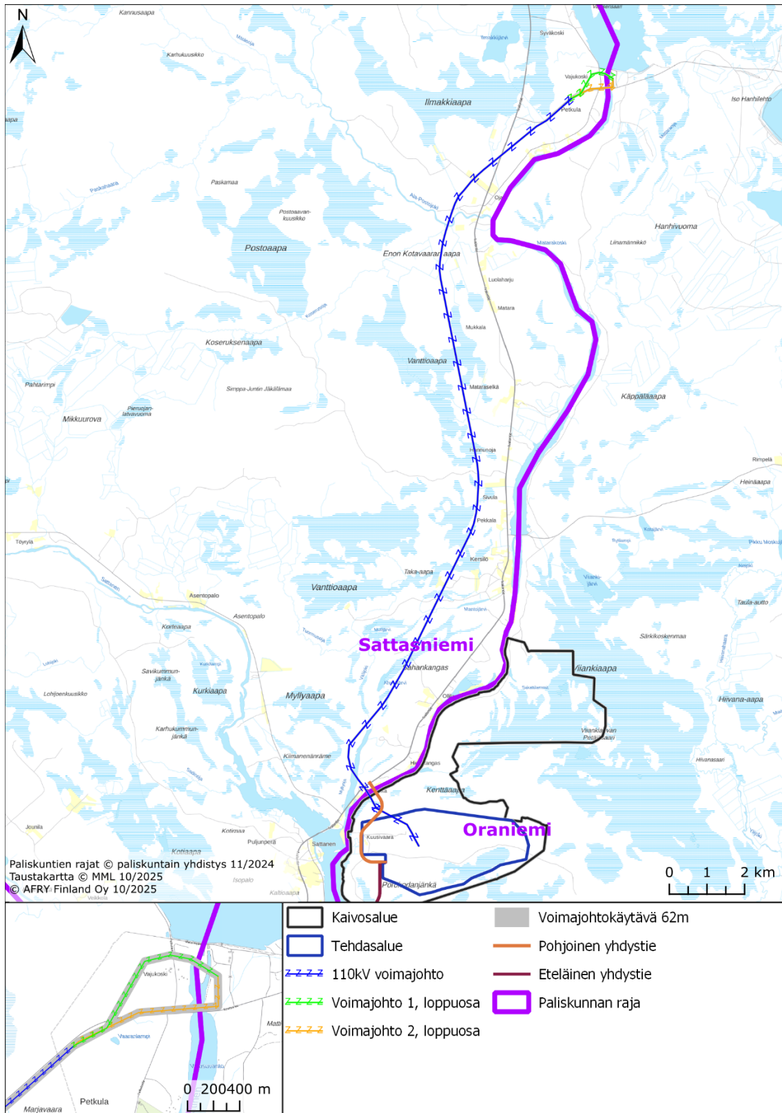
Kuva 2-2. Sakatin kaivoshankkeen suunniteltu voimajohto hankkeen sähkönsiirtoon.
