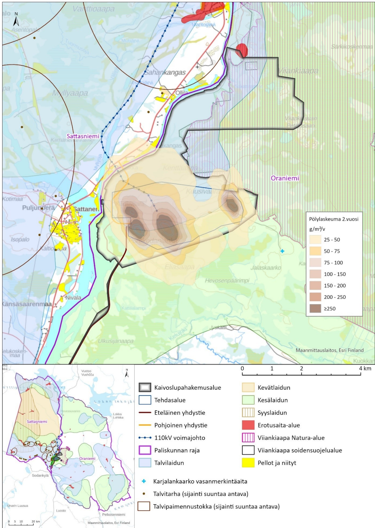
Kuva 5-5. Pölypäästön leviäminen 2. toimintavuonna kun rikastushiekka-aluetta rakennetaan ja tarvekilouhoksen toiminta on alkanut.
