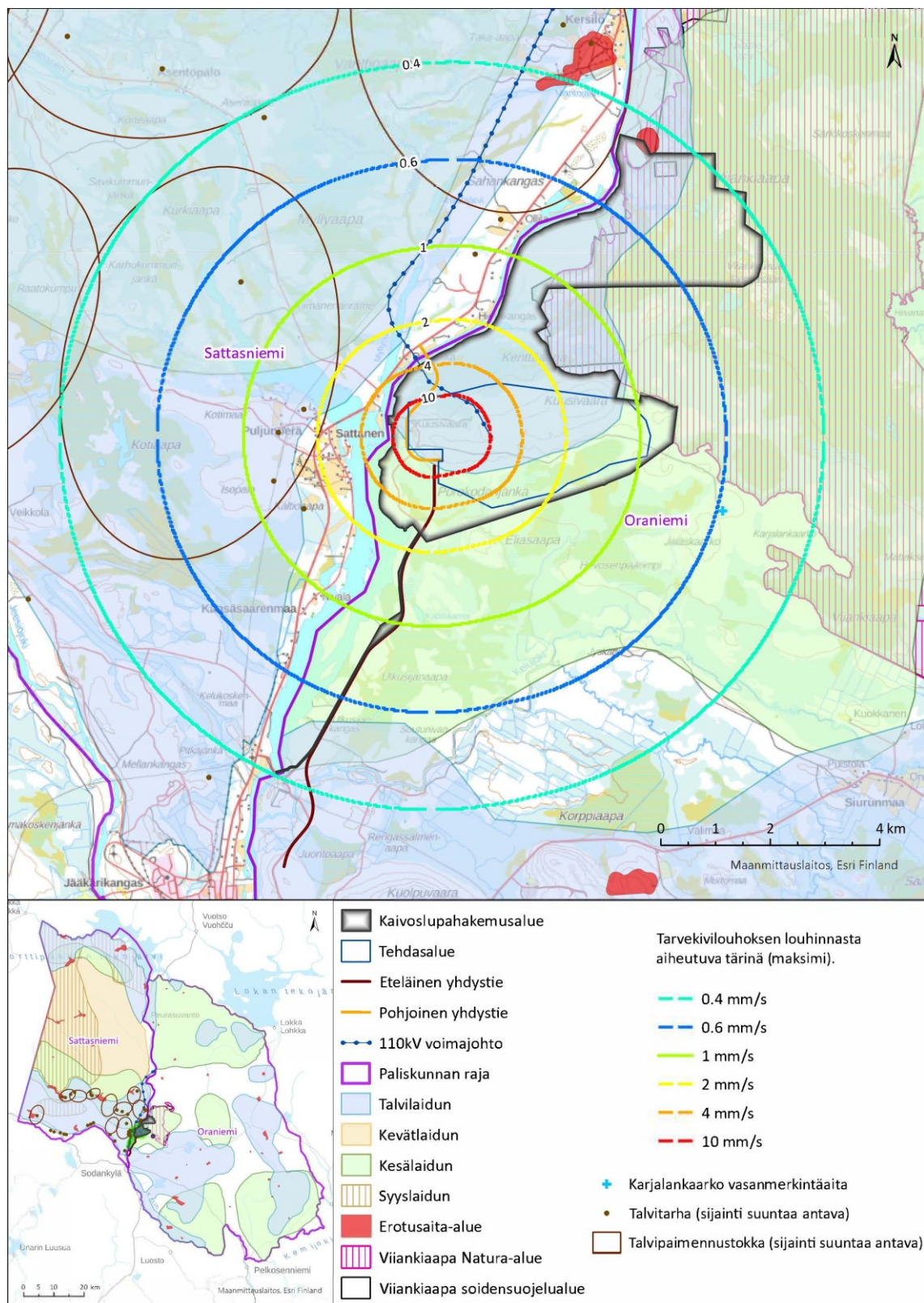
Kuva 5-4. Tarvekilouhoksen louhinnasta aiheutuva värinän leviämisalue (maksimi), kun tarvekiveä louhitaan vaiheessa 3.
