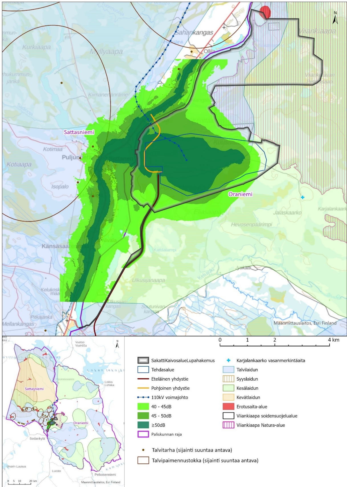
Kuva 5-8. Toiminnan aikainen melu maksimitilanteessa tuotantovaiheessa 2. Mallinnuksessa on huomioitu vt 4 liikenteestä aiheutuva päiväaikainen melu (L Aeq PÄIVÄ 07-22).
