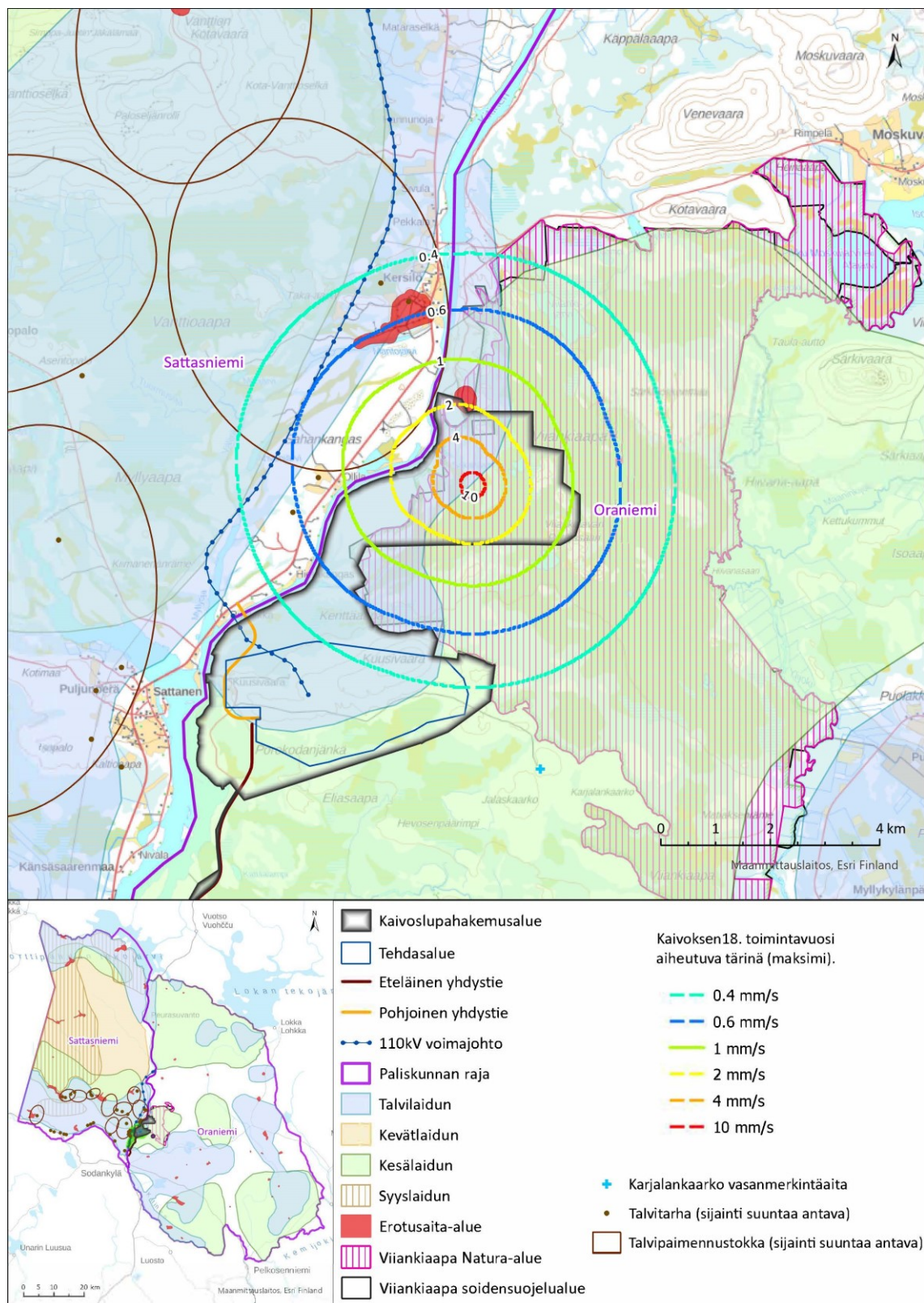
Kuva 5-9. Tärinän leviämisen laajin mahdollinen tilanne maanalaista louhintaa tehtäessä toimintavuonna 18.
