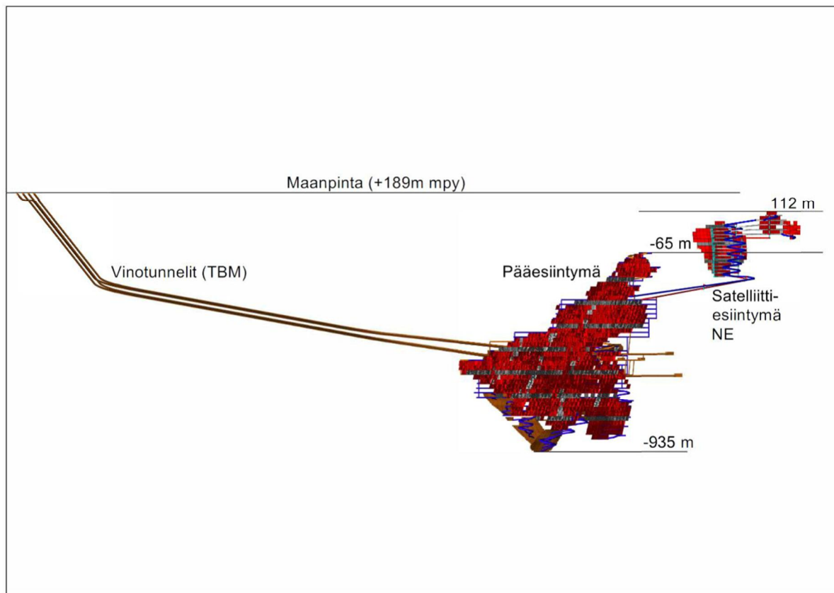
Kuva 4. Pituusleikkauskuva Sakatin maanalaisesta kaivoksesta. Sakatin pääesiintymän ylin louhintataso sijoittuu 65 metriä merenpinnan eli noin 250 metriä maanpinnan tasosta. Satelliittiesiintymän NE ylin louhintataso sijoittuisi noin 112 metriä merenpinnan yläpuolella, eli noin 80 metriä maanpinnan tasosta.
